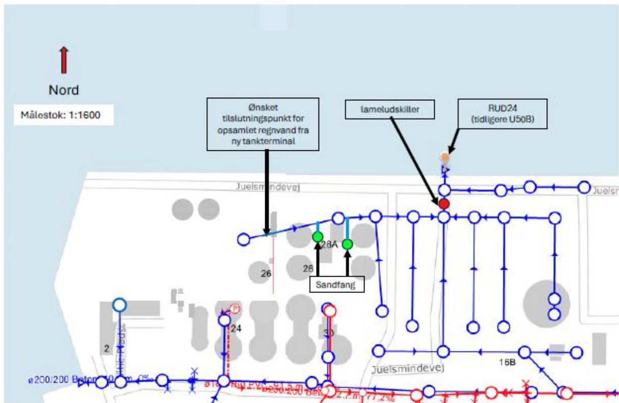
Figur 2: Situationsplan som viser tankgården ved Juelsmindevej, 4400 Kalundborg. Planen var en del af det indsendte ansøgningsmateriale og er ikke målfast.
