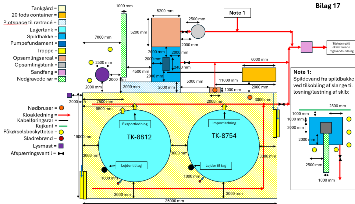
Figur 3: Overblik over forskellige spildebakker og opsamlingstanke
