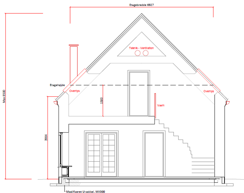
4 – Principsnit af det ansøgte.
