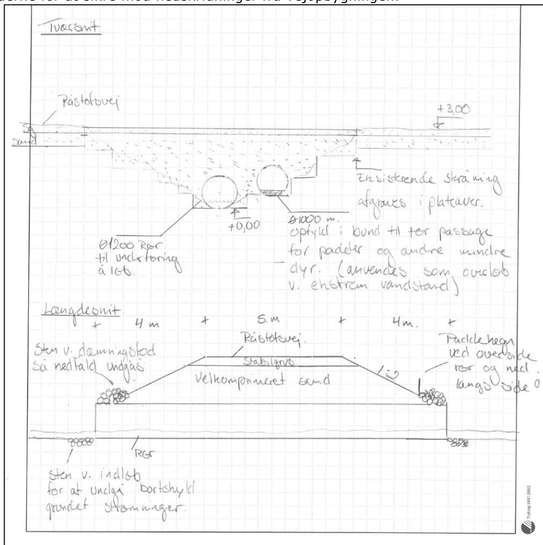
Figur 3: Skitsetegning i tværsnit og længdesnit af røroverkørsel. Udklip fra Ansøgning om råstofvej samt lovliggørelse af adgange til Kaldredvej af 20. juni 2025 , udarbejdet af Colas Danmark A/S, Meteorvej 16, 8700 Horsens.
