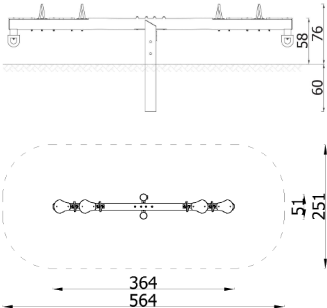
6 – Specifikke mål for den ansøgte vippe.
