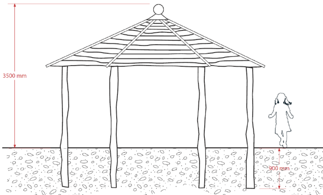
3 – Facadetegning af det ansøgte madpakkehus.
