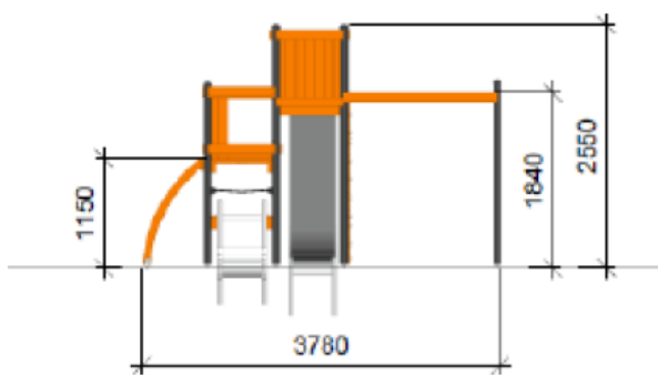
2 - Tegning af det ansøgte klatrestativ.
