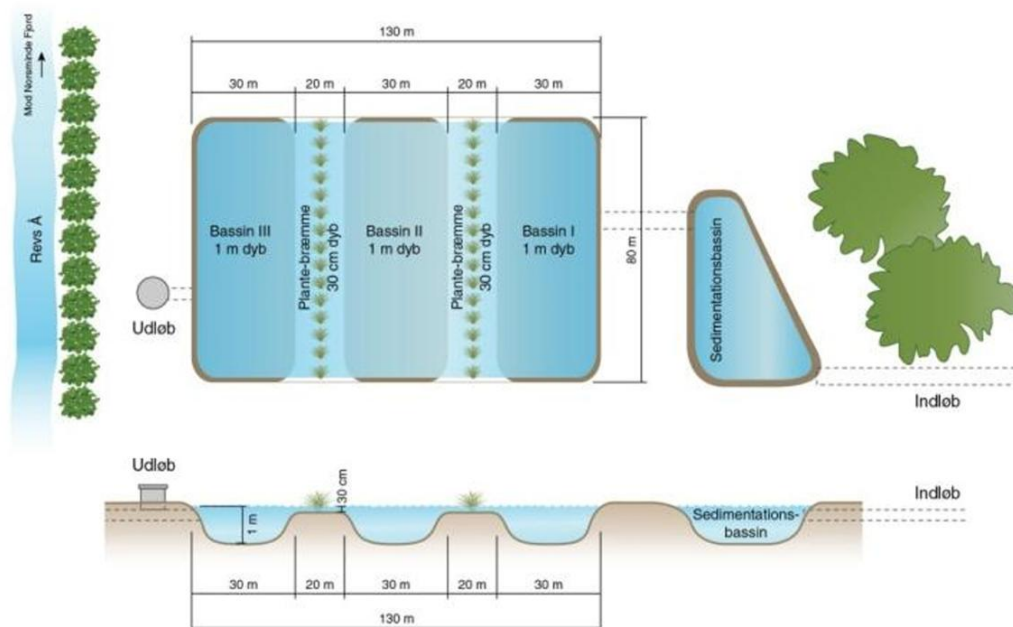
Principskitse af design af minivådområde (Kjærgaard, C. 2023)
